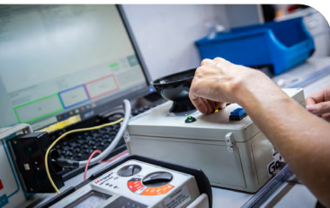
Testování relétek.
